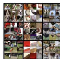
Layer 4
