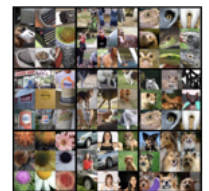
Layer 5
