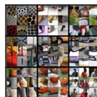
Layer 3
